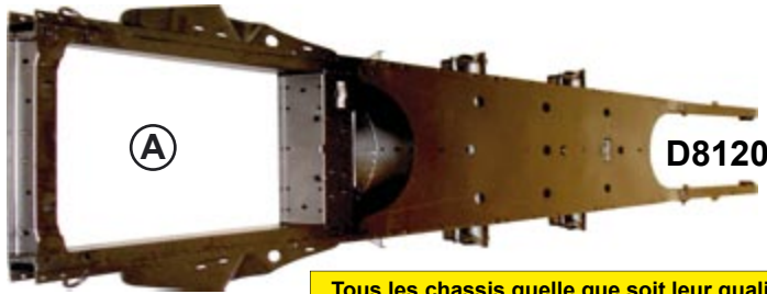
Chassis Noir Traitement par Electrozinguage + Cataphorèse Top Qualité
